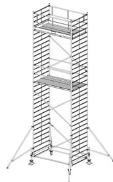
Arbeitshöhe: 9,40 m Gerüsthöhe: 8,40 m Standhöhe: 7,40 m
