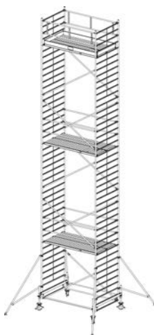
Arbeitshöhe: 12,40 m Gerüsthöhe: 11,40 m Standhöhe: 10,40 m
