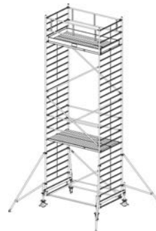
Arbeitshöhe: 8,40 m Gerüsthöhe: 7,40 m Standhöhe: 6,40 m
