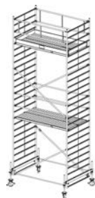
Arbeitshöhe: 7,40 m Gerüsthöhe: 6,40 m Standhöhe: 5,40 m
