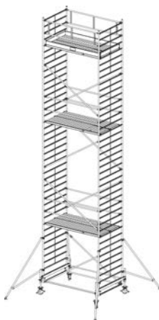
Arbeitshöhe: 11,40 m Gerüsthöhe: 10,40 m Standhöhe: 9,40 m
