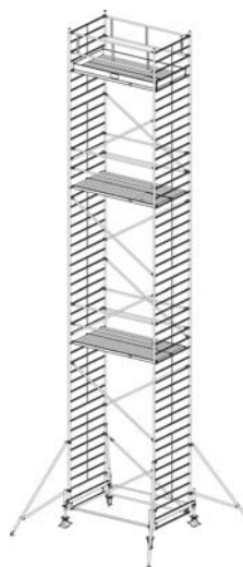
Arbeitshöhe: 13,40 m Gerüsthöhe: 12,40 m Standhöhe: 11,40 m
