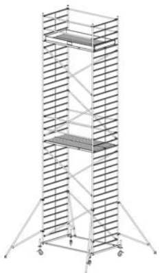
Arbeitshöhe: 10,40 m Gerüsthöhe: 9,40 m Standhöhe: 8,40 m
